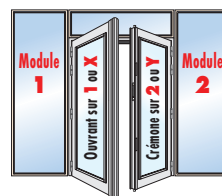
Façade n°211 Avec porte : croquis 6
