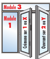
Façade n°308 Avec porte : croquis 6
