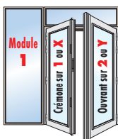
Façade n°208 Avec porte : croquis 6
